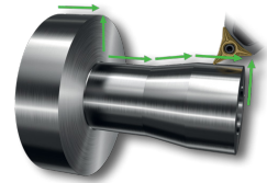
PrimeTurning™
