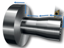
konventionelles Drehen
