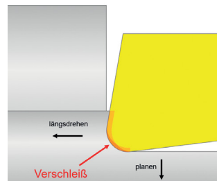
konventionelles Drehen
